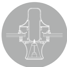
Sparren-Variante AUSSENLIEGENDER SPARREN mit Leuchtenkanal
