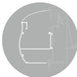
Rinnen-Variante RUNDES PROFIL
