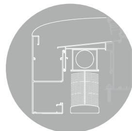
Rinnen-Variante GERADES PROFIL mit versenkbarem Raffstore
